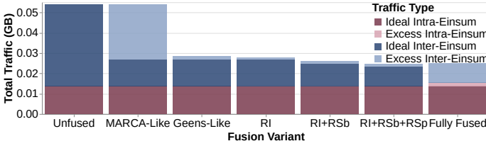
(a) Prefill phase (B=64, I=2048).
