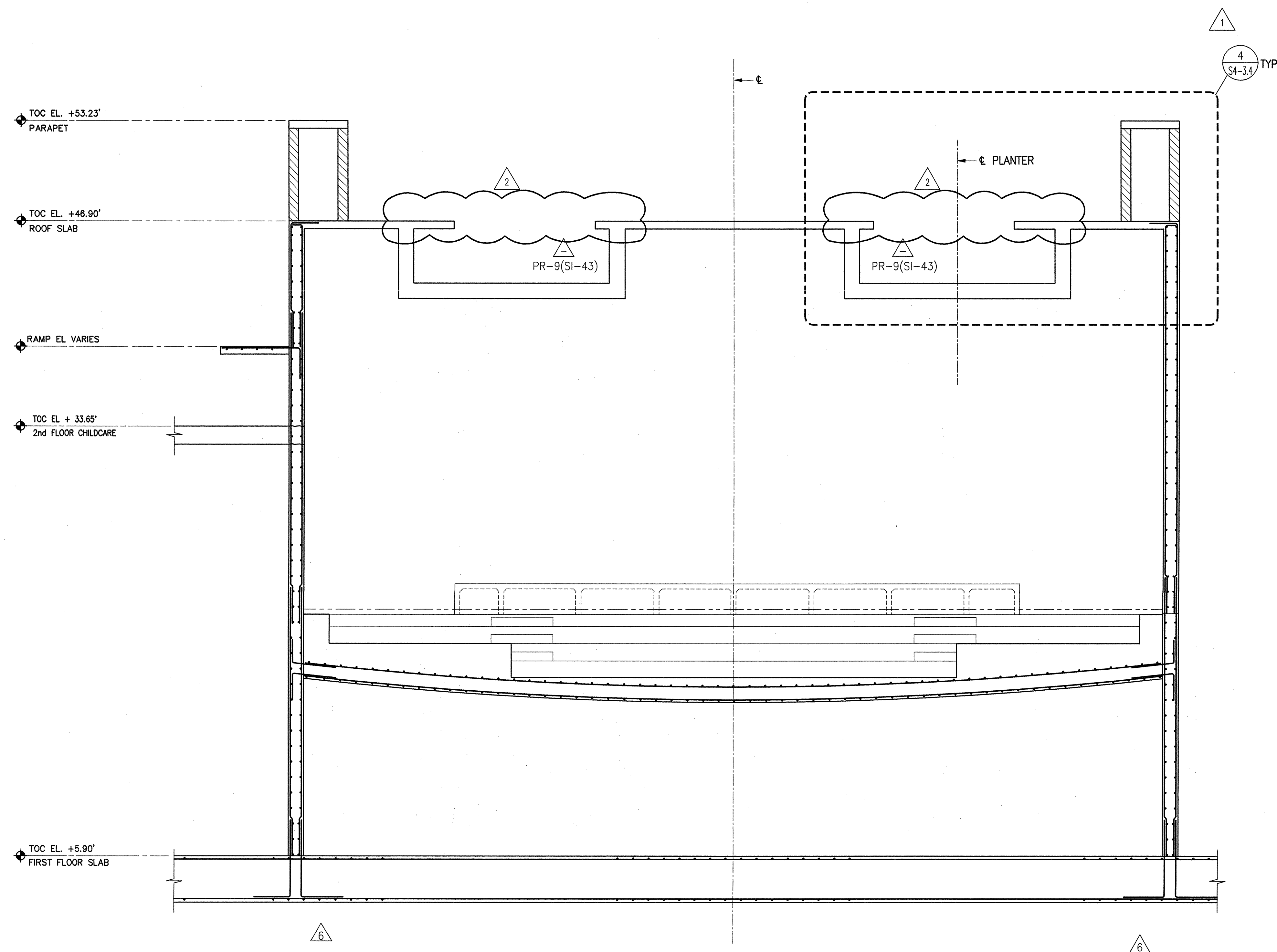
3 SECTION • PLANTER 1/4"=1'-0"
