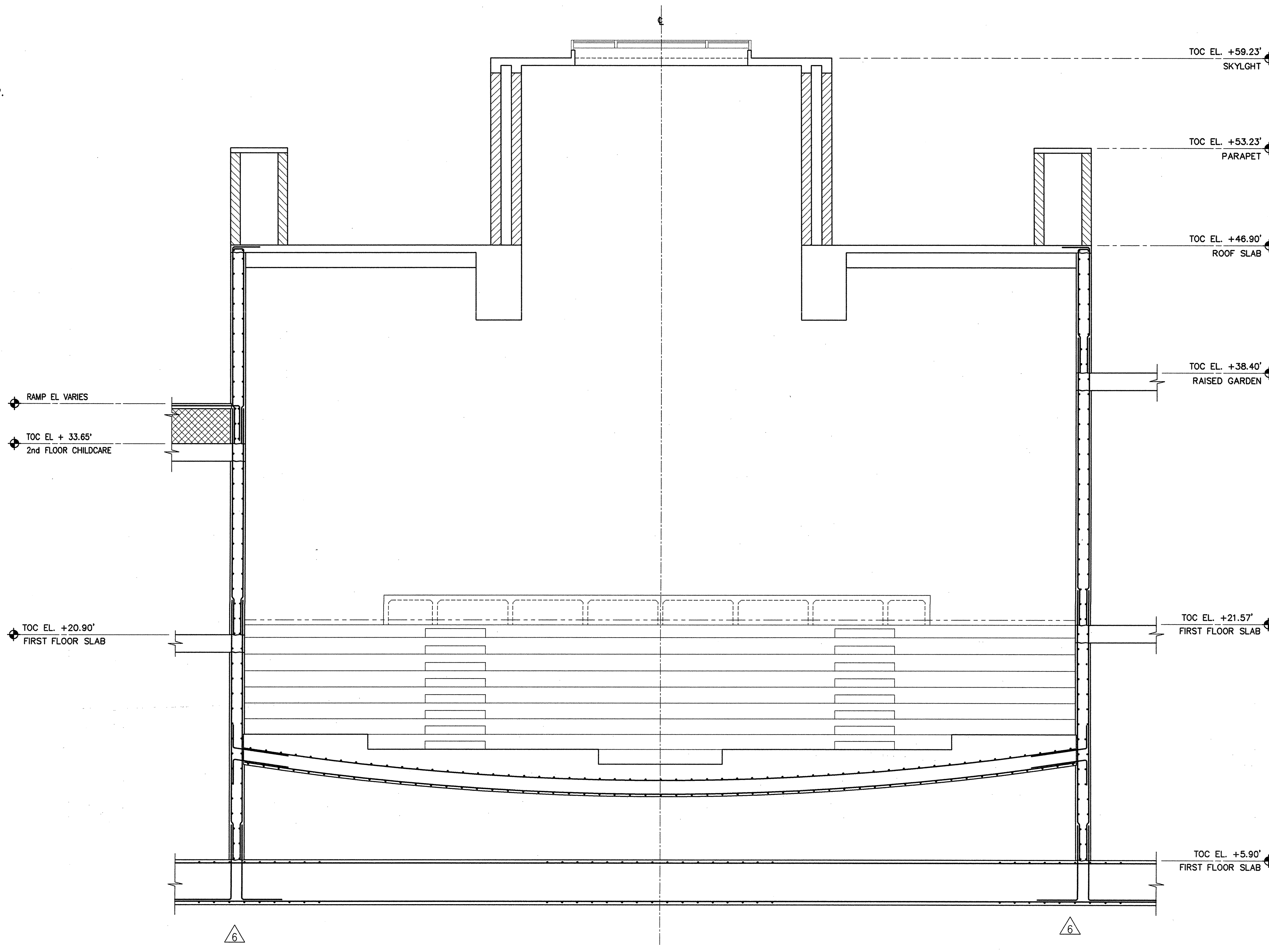
1 SECTION • CENTER 1/4"=1'-0"
